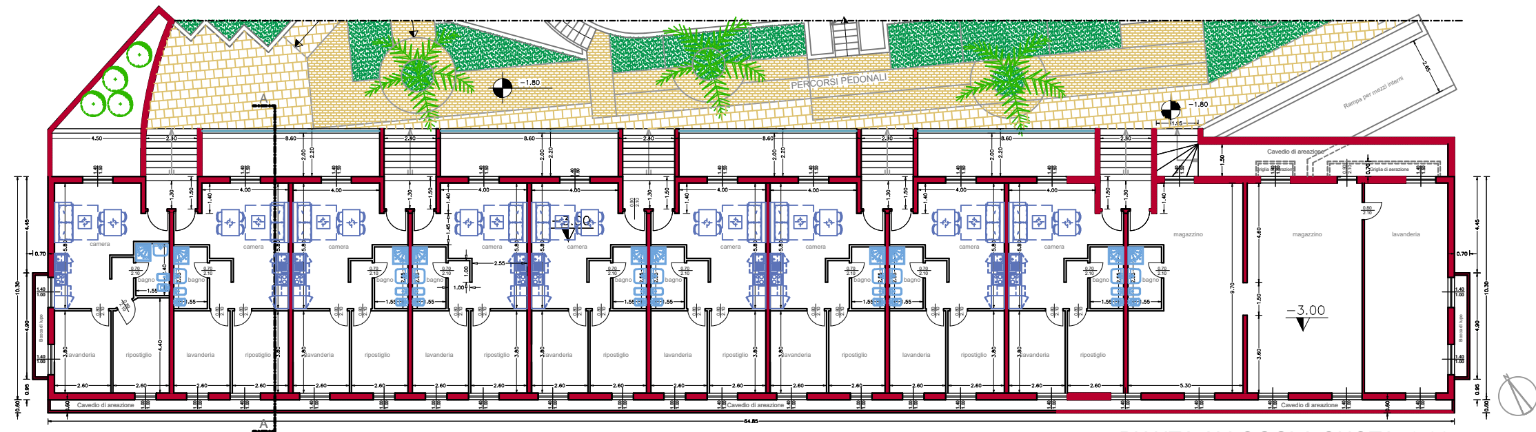
PIANTA ALLOGGI A QUOTA -3.00
