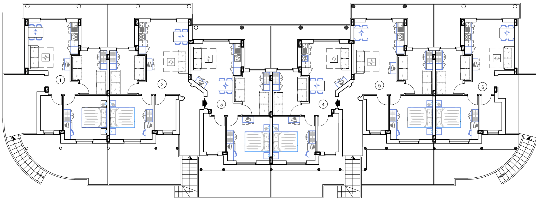
PIANTA PIANO PRIMO BLOCCO CAMERE DA N.3
